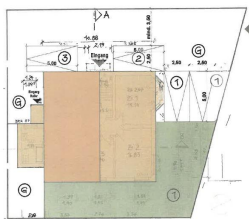
L. Baumbach Baugesellschaft mbH 37133 Friedland LAGEPLAN M 1:425
